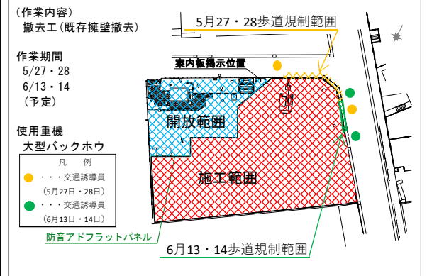
歩道規制範囲平面図
