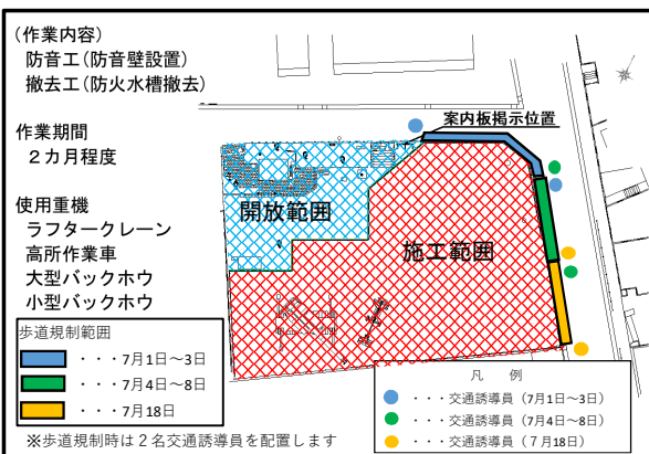
歩道規制範囲平面図
