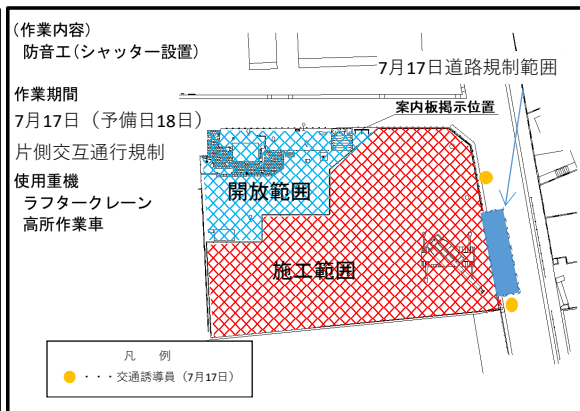
道路規制範囲平面図
