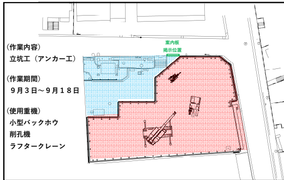
工事規制範囲：ステップ3-1
