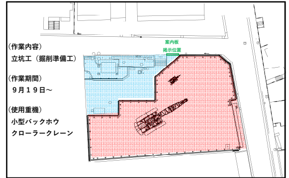
工事規制範囲：ステップ3-2
