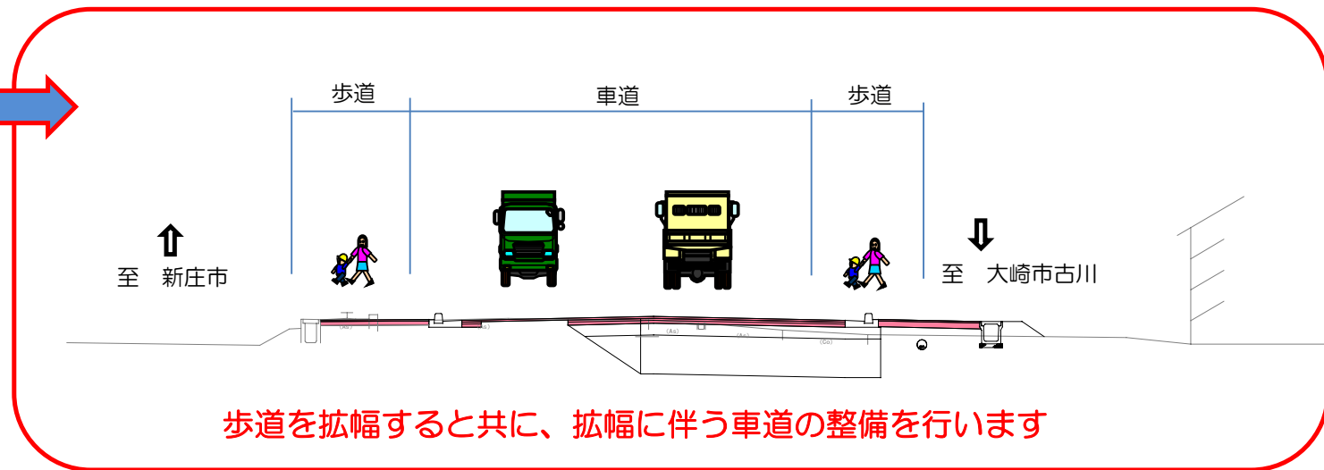
〔標準横断 完成図〕
